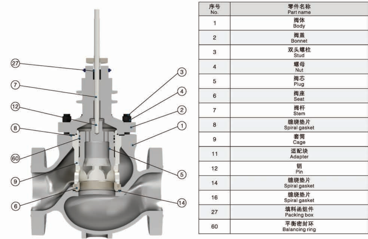
◆图1 标准套筒调节阀本体部结构图 Fig. 1 Structure of standard sleeve control valve
